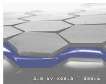
異形 Si チップのダイシング例 (グラインド後)
