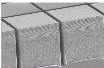
ダイシング例 (グラインド前)
