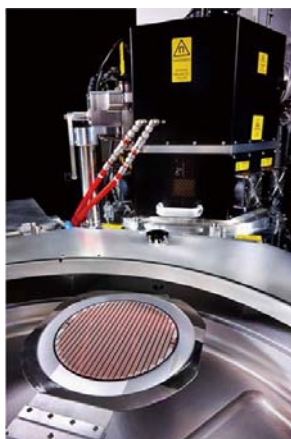
Mosaic fxP の装置外観
